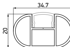
F40 Classic vertikalni profil 20×34.7 mm - 6 m Antracit RAL 7016
