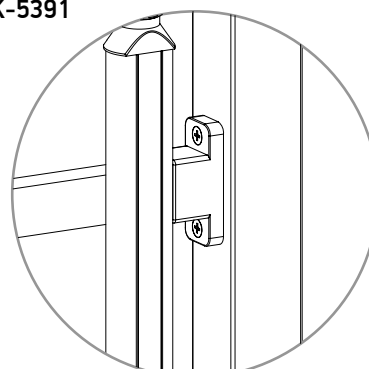
Detalj B
