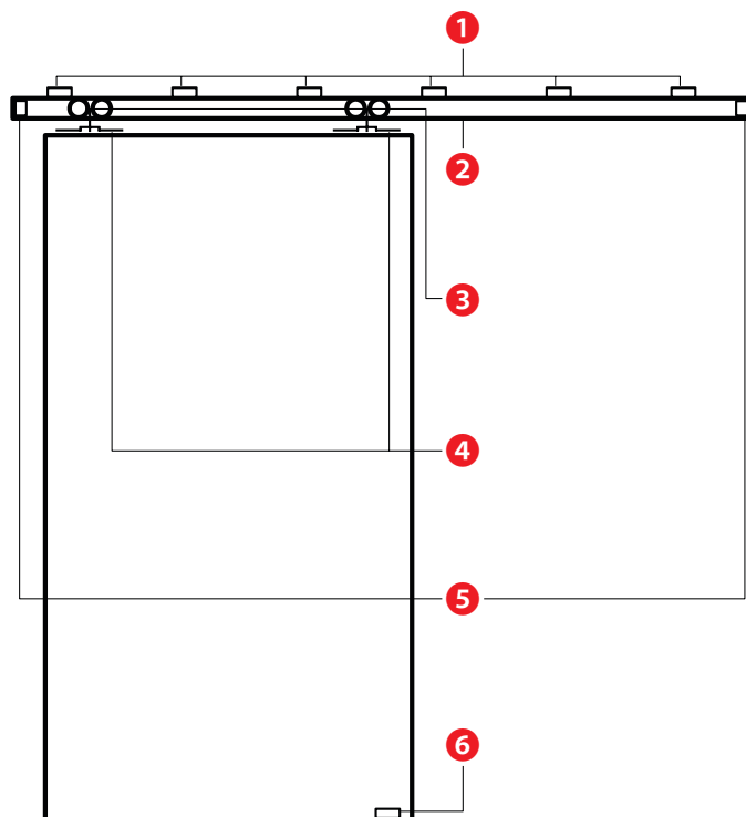
Šema montaže za drveno krilo
