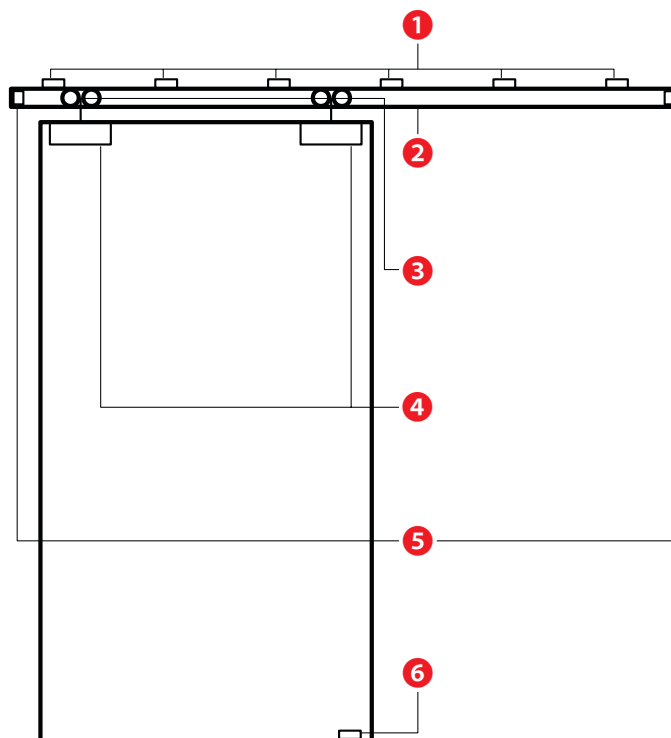
Šema montaže za stakleno krilo
