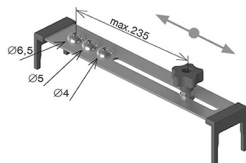
Šablon za bušenje Ø42.4x2mm, 40x40x2mm
