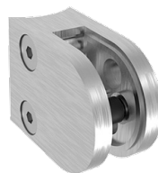
Inox nosač za stub Ø42.4 staklo 6-10.76 mm AISI 316 - Satinirano
