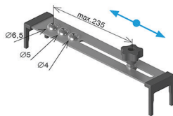
Šablon za bušenje Ø42.4x2mm, 40x40x2mm A/40580-PLASTIC 44.00€
