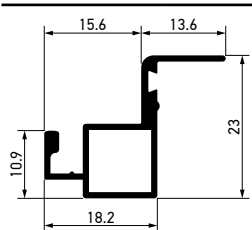
Profil 23 mm za fiksni komarnik Lux - Bela 9016 - 6 m
