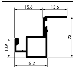
Profil 23 mm za fiksni komarnik Lux - Antracit 7016 - 6 m
