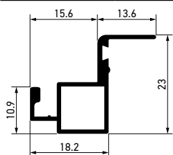
Profil 23 mm za fiksni komarnik Lux - Sirovo - 6 m
