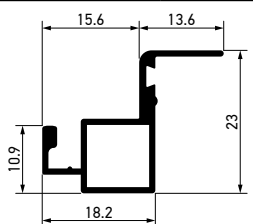
Profil 23 mm za fiksni komarnik Lux - Zlatni hrast - 6 m
