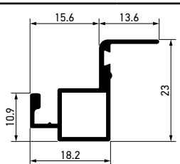
Profil 23 mm za fiksni komarnik Lux - Crna 9005 - 6 m
