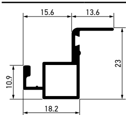
Profil 23 mm za fiksni komarnik Lux - Braon 8014 - 6 m
