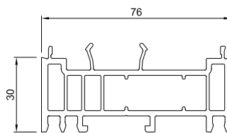
Proširenje 76×30 mm
