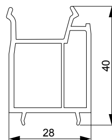
Podštok 28×40 mm
