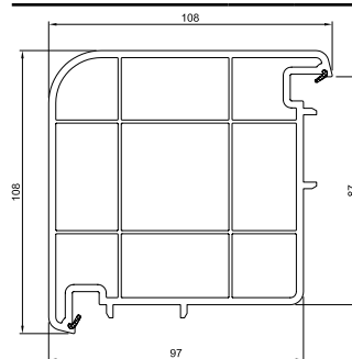
Skretnica 90° 76 mm
