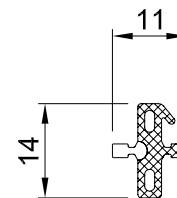
Spoj štokova
