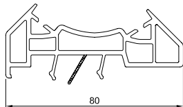
Adapter za varijabilnu skretnicu
