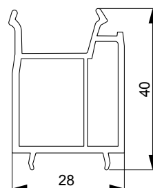
Podštok 28×40 mm
