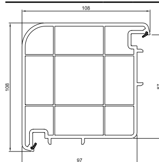
Skretnica 90° 76 mm
