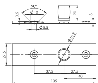
3 Plafonski prihvatak gornje figure - AISI 304 GS-304/ZP802/S 5.22€
