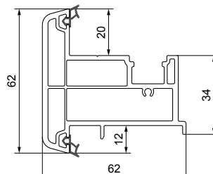
Lažna prečka 62 mm
