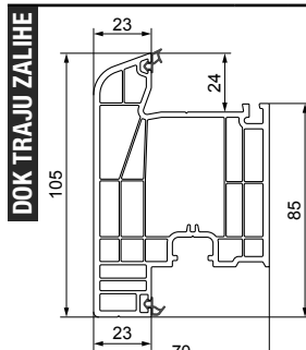
Krilo vrata - 70 mm
