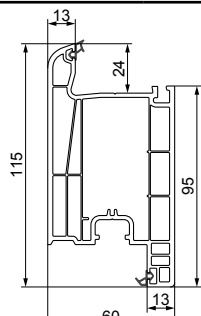
Krilo vrata - 60 mm
