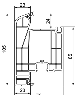
Krilo vrata - 70 mm
