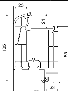
Krilo vrata - 70 mm
