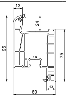
Krilo balkonca - 60 mm
