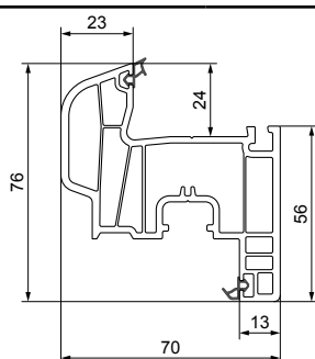
Krilo sa 5 komora
