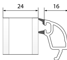
Lajsna za staklo 24 mm
