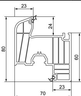
Krilo sa 6 komora - 70 mm
